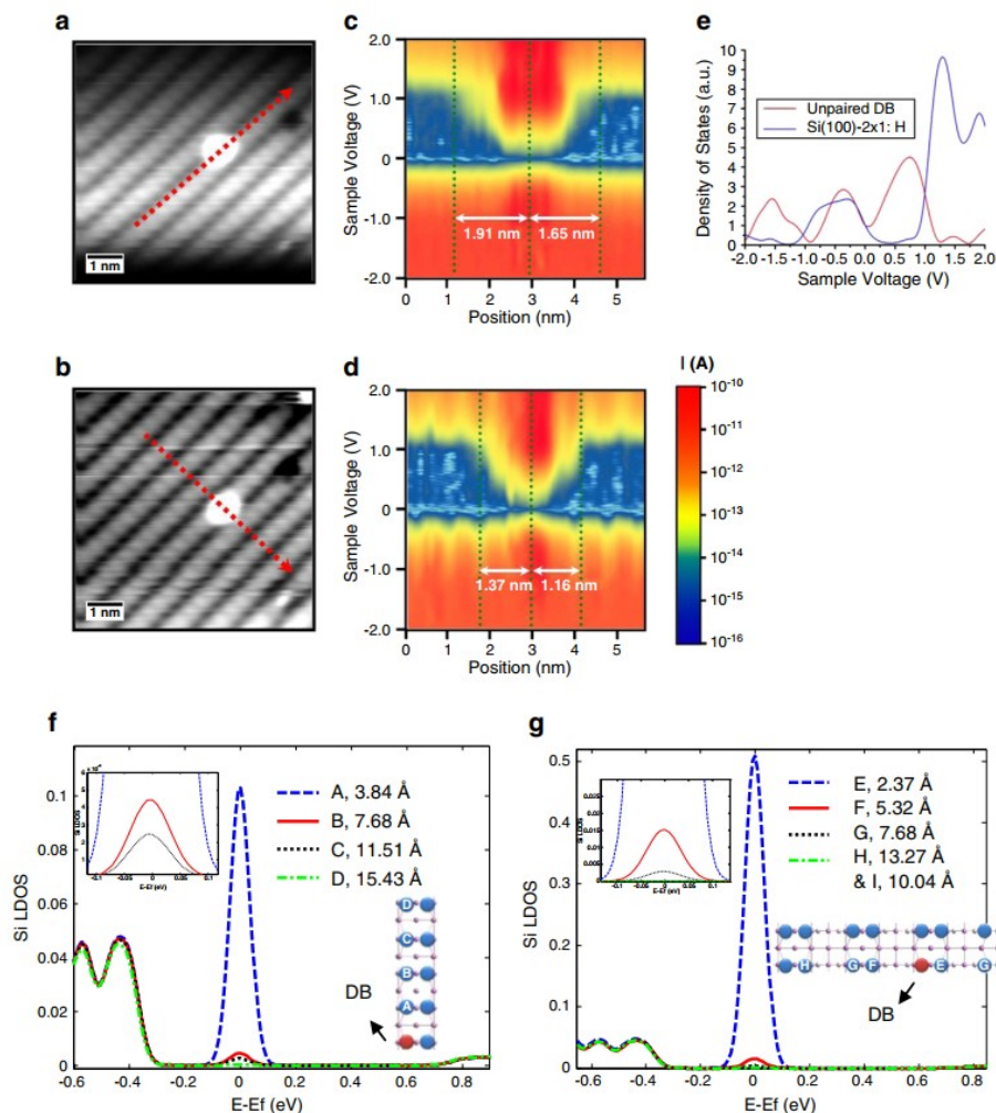
Рис. 4. (а) STM-изображение непарной оборванной связи в заполненном состоянии на поверхности Si(100)-2×1:H. ( V_s=-2,0 В, I_t=50 Па) (б) STM-изображение БД в том же димере Si после переключения положения слева направо. (с, d) Логарифмические спектры I–V, построенные в зависимости от положения в (с) для непарного ОС в (а) и в (d) для ОС в (б). Красные пунктирные стрелки в (а) и (б) указывают, где были получены карты I-V спектров. Зеленые пунктирные линии в (с) и (d) используются для выделения положений центра непарного ОС и где ширина запрещенной зоны Si полностью равна восстановленный. (е) спектры DOS-V непарного ОС в (а) и кремниевой подложке. (f) Смоделированные LDOS атомов Si вдоль направления димера Si с расстоянием от ОС. (Вставка показывает увеличенный вид для атомов B, C и D.) (g) Смоделированные LDOS атомов Si в направлении димера Si с расстоянием от ОС. (Вставка показывает увеличенный вид атомов F, G, H и I.).
