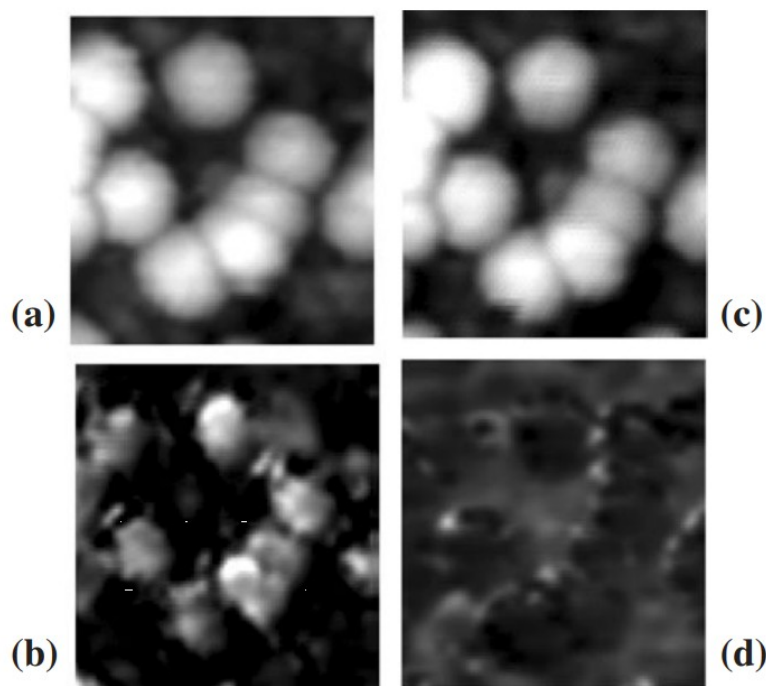
Рис. 2. STM топографии поверхности окисленного Si(100)-(2 × 1) толщиной ≈0,3 нм до (а) и после осаждения кластеров C 60 (б) и Si 6 H x (в). Плотность скоплений составила ≈3 × 10 12 см -2 в (с) и ≈2 × 10 13 см -2 в (б). Области изображения составляют 50 × 50 нм 2 в (а) и (б) и 50 × 30 нм 2 в (с). На вставке (а) показана поверхность Si(100)-(2 × 1) площадью 20 × 20 нм 2 , полученная после мгновенного нагрева при 1100°С. Начальное напряжение составляло +2 В, а туннельный ток составлял 0,3 нА.
