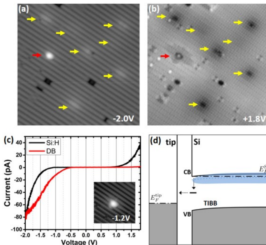
Рис. 7. (20 \times 20) нм 2 при постоянном токе (30 пА) заполненное состояние (а) и пустое состояние (б) STM-изображения поверхности Si(100): Н - 2 \times 1 образца, обработанного вспышкой при 1050°C. Желтые стрелки указывают на подповерхностные примеси (As), в то время как красная стрелка указывает на единственный DB. (с) I(V) спектроскопия, полученная на единичном DB (красная кривая) и поверхности Si:H (черная кривая). Вставка на (с) показывает изображение STM с постоянным током, на котором одиночный DB выглядит ярким при -1:2 В. (d) Схематическая диаграмма энергетического диапазона, показывающая механизм туннелирования через DB в случае высоколегированного образца при 1050°C. Штрих-пунктирные линии представляют уровни Ферми наконечника и образца, E_F^{tip}; Si . Заштрихованная синяя область указывает на образование донорной полосы, которая сливается с зоной проводимости.
