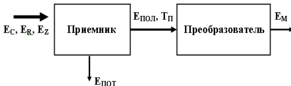
Рис.1. Схема солнечных теплоэнергетических установок.
