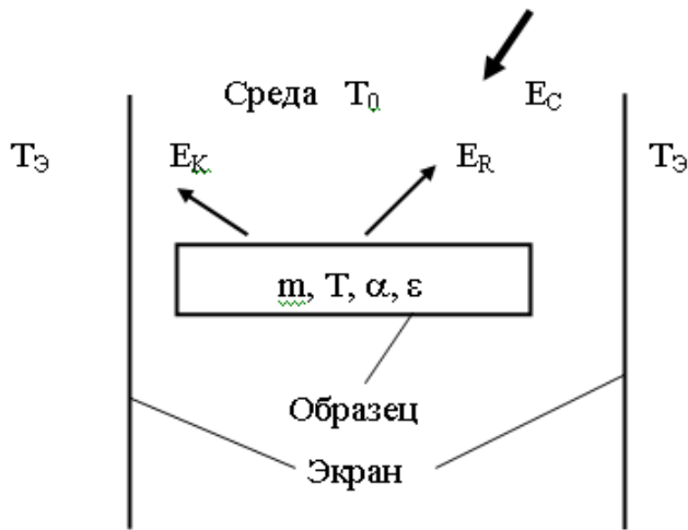
Рис.2. Схема определения излучательной способности прямыми методами.
