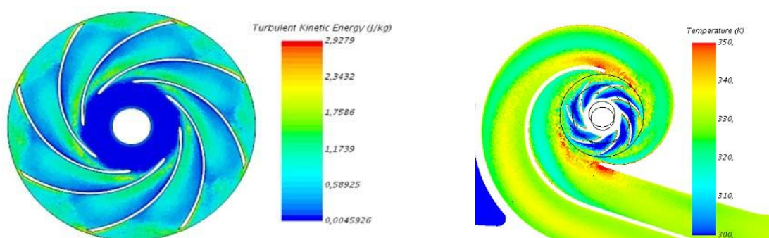
Рисунок 2. Распределение турбулентной кинетической энергии в рабочем колесе насоса ( ns=34 ) и температуры в насосе двустороннего входа ( ns=234 )
