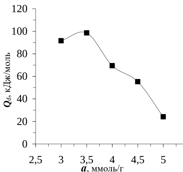
Рис.3. Зависимость дифференциальных изостерических теплот ( Q_d ) адсорбции \text{CH}_3\text{SH} в цеолите NaX от адсорбции ( a ).
