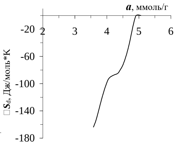
Рис.4. Зависимость дифференциальной энтропии ( \Delta S_d ) адсорбции \text{CH}_3\text{SH} в цеолите NaX от адсорбции ( a ). Энтропия жидкого \text{CH}_3\text{SH} принята за ноль.
