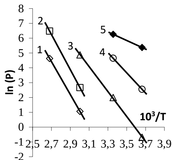
Рис.2. Зависимость логарифма давления ( \ln P ) \text{CH}_3\text{SH} в цеолите NaX от обратной температуры ( 10^3/T ), соответствующая различным количествам адсорбированного вещества (ммоль/г): 1 - 3,0; 2 - 3,5; 3 - 4,0; 4 - 4,5; 5 - 5,0.
