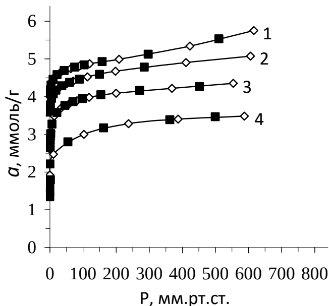
Рис.1. Зависимость адсорбции ( a ) \text{CH}_3\text{SH} в цеолите NaX от давления ( P ): 1 – 273 К; 2 – 298 К; 3 – 333 К; 4 – 373 К. Черные точки рассчитаны с помощью уравнения ТОЗМ.
